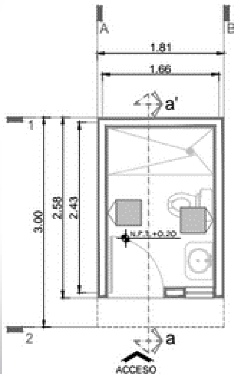
PLANTA ARQUITECTÓNICA BAÑO
